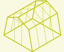
SERRES À PAROIS OBLIQUES voir p.14 et p.33 pour toutes les dimensions
